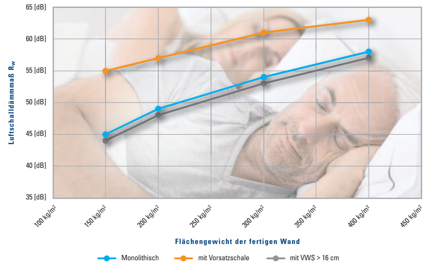
Luftschalldämmmaß R_w massiver Wände in Abhängigkeit vom Flächengewicht der Gesamtkonstruktion
